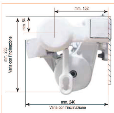
Attacco parete
