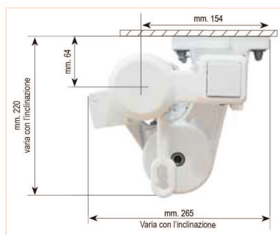
Attacco soffitto
